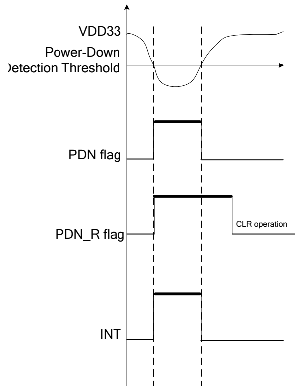
图 5-2 掉电中断
