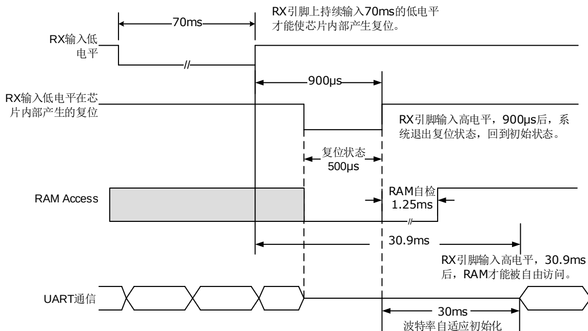
图 2-1 RX 复位时序图
