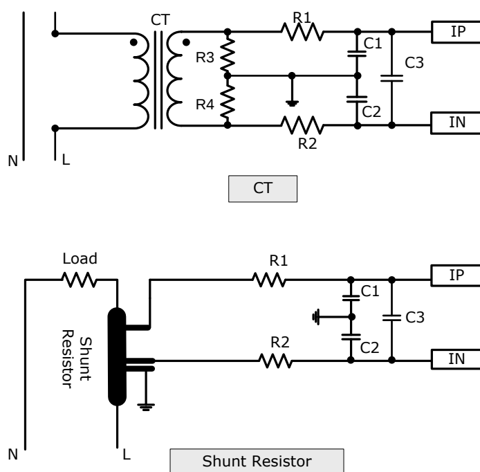
图 8-1 电流输入方式
