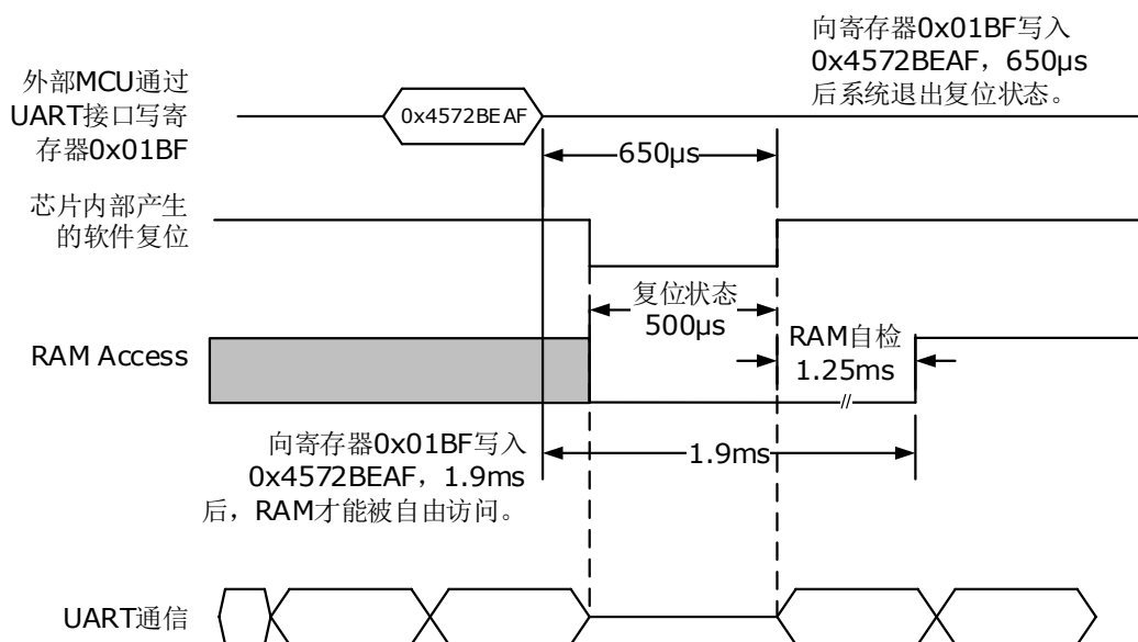
图 2-2 软件复位时序图
