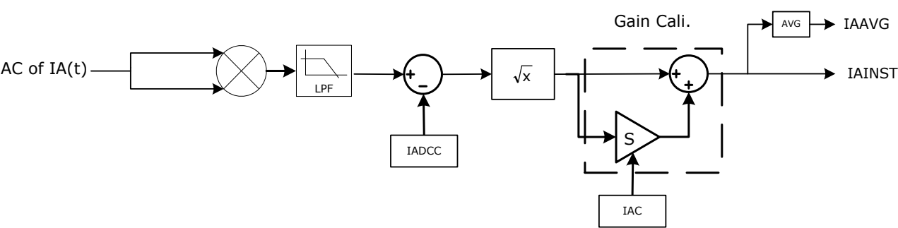
图 8-5 有效值信号处理
