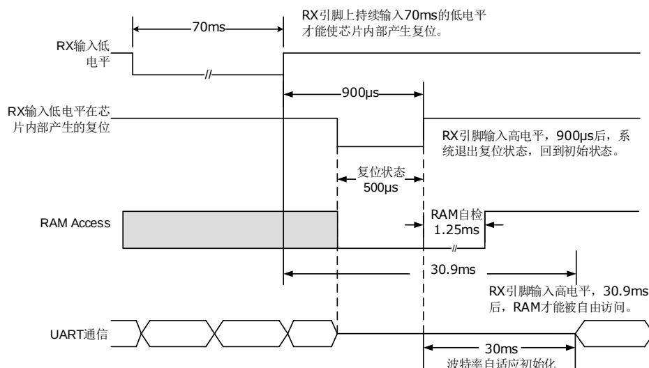
图 2-1 RX 复位时序图
