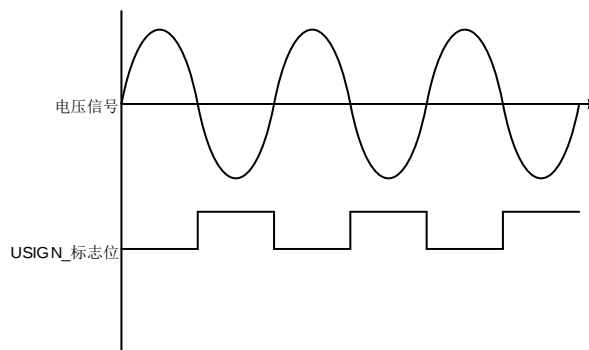
图 9-1 电压过零点中断
