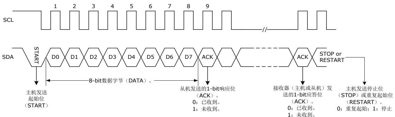
图 15-1 通信帧结构
