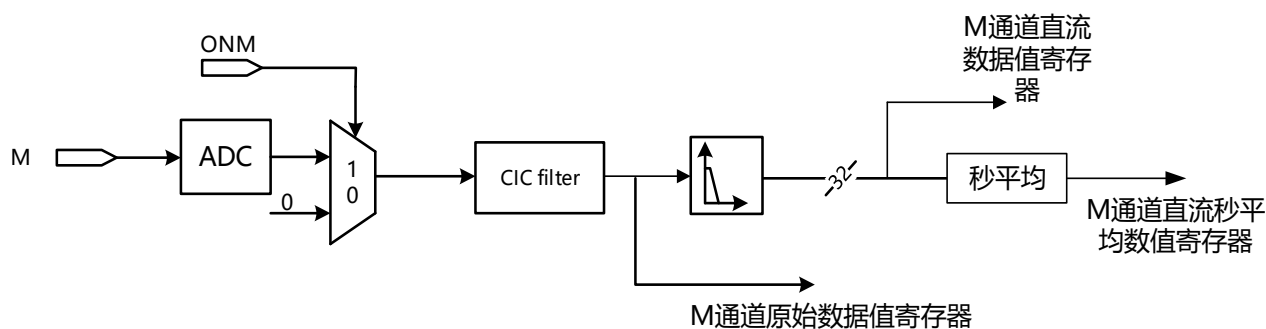
图 11-15 M 通道内部连接图
