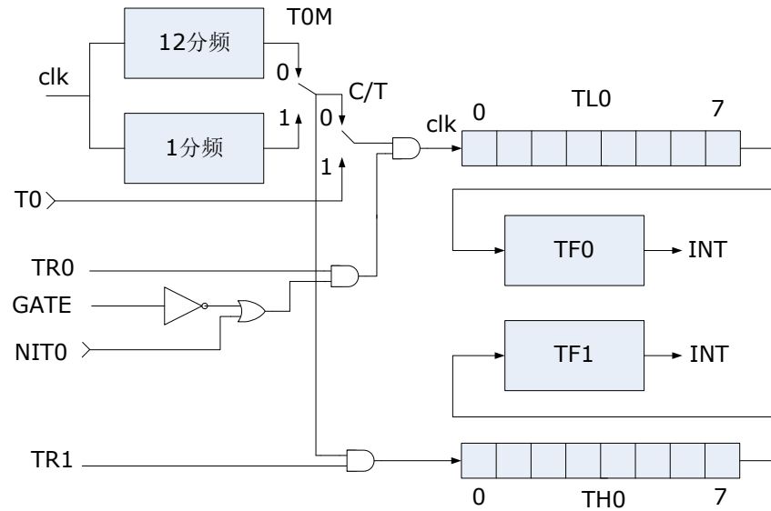
图 14-9 Timer0/1 模式 3
