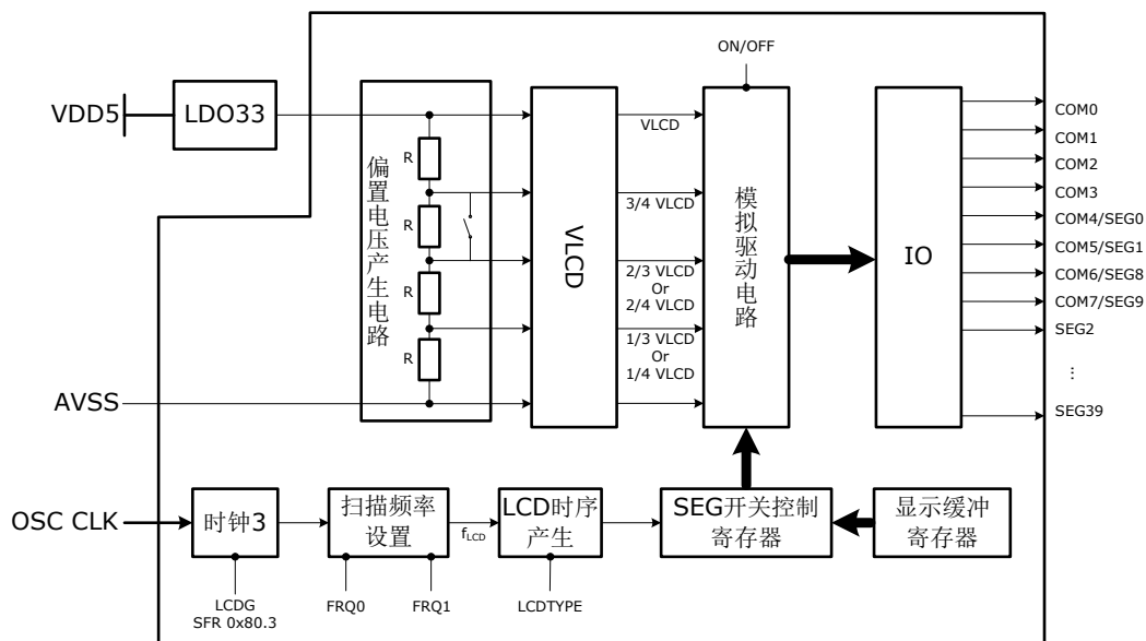
图 16-1 LCD 驱动电路结构图
