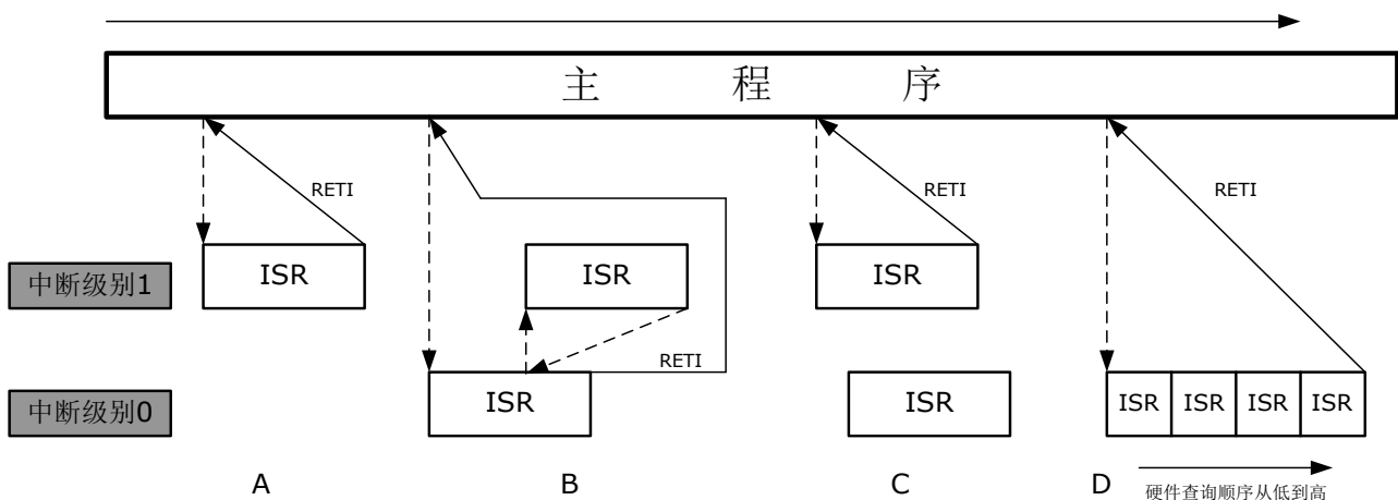
图 13-2 中断处理
