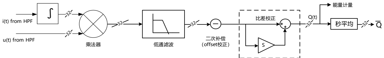
图 11-11 无功功率计算
