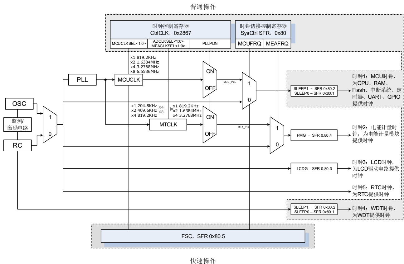
图 9-1 时钟控制电路框图
