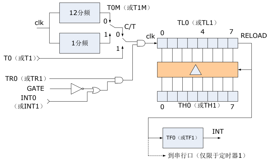
图 14-8 Timer0/1 模式 2
