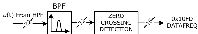
图 11-13 线电压频率测量原理
